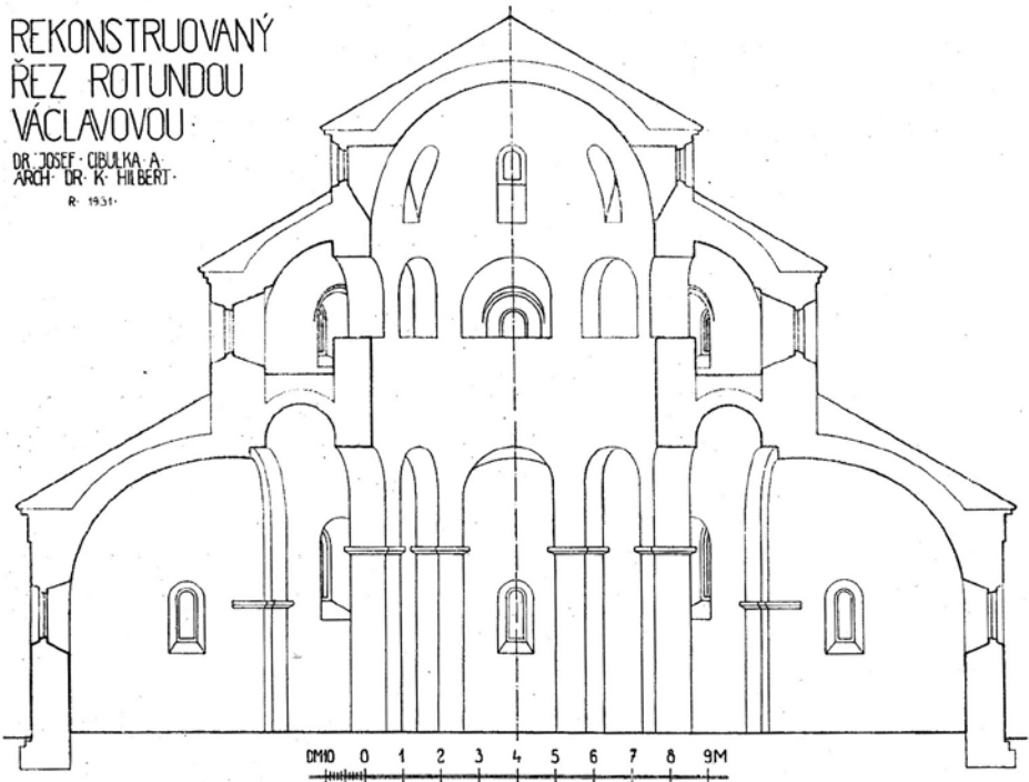
Rekonstrukce rotundy v řezu (podle J. Cibulky a K. Hilberta)
